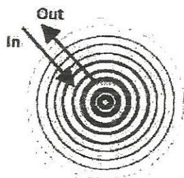
Εικόνα 5: Η ύπαρξη ενός σωματιδίου φυσικής ύλης είναι εξαρτώμενη από την αλληλεπίδραση δια μέσω κβαντικών κυμάτων με όλα τα άλλα σωματίδια στο σύμπαν.
