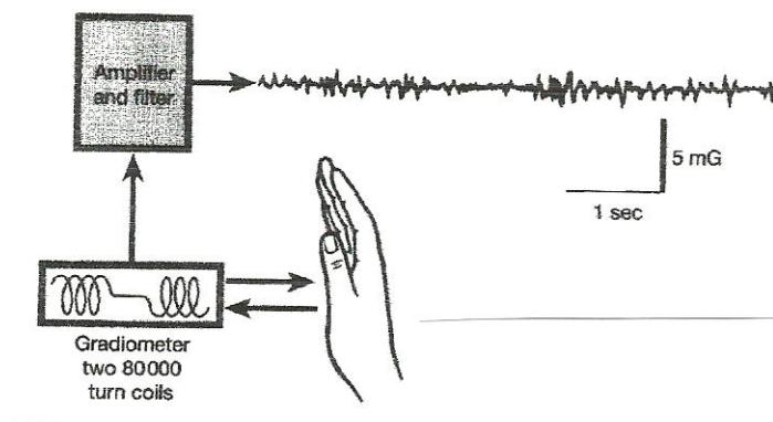
Εικόνα 3: Παλλόμενα βιομαγνητικά πεδία τα οποία μετρούνται κατά τη διάρκεια εκπομπών Κί (Seto, 1992)
